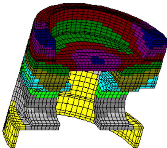
Рис. 6 Вид КОНСТРУКЦИИ при Lbrv=0,1
