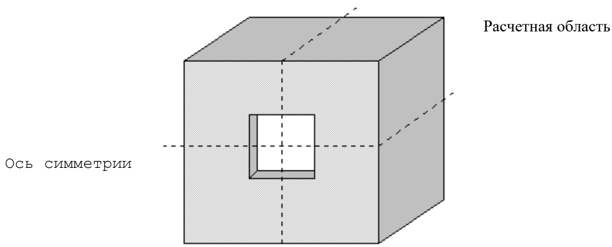
Рис.8. Выбор расчетной области
