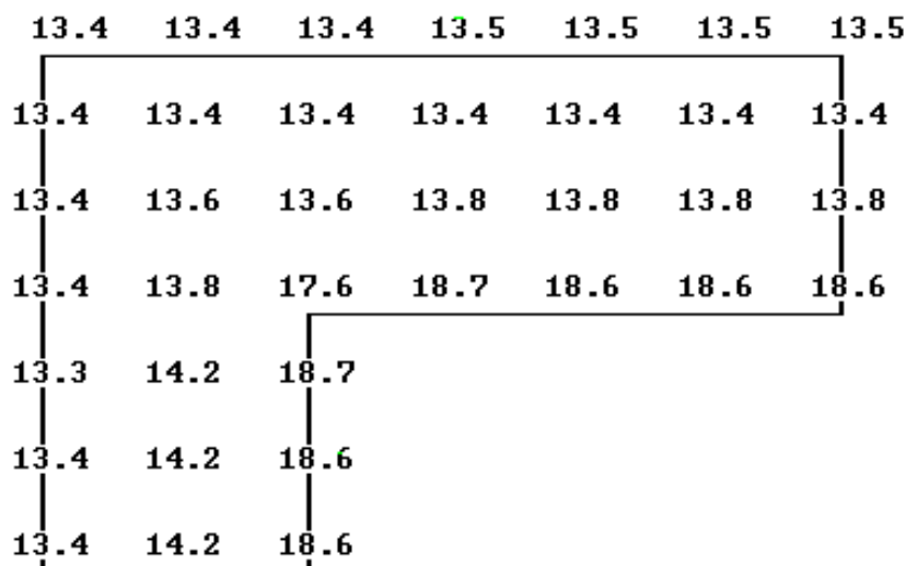
Рис.13. Температурное поле внутренней поверхности в режиме "Псевдографика", (пример test1).
