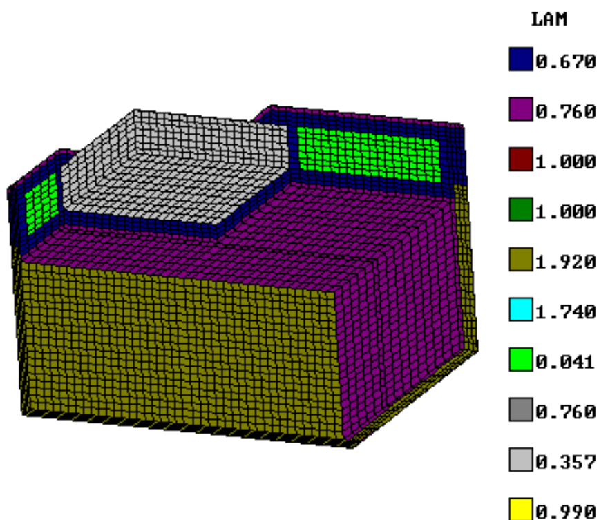
Рис.10. Задание характеристик материалов
