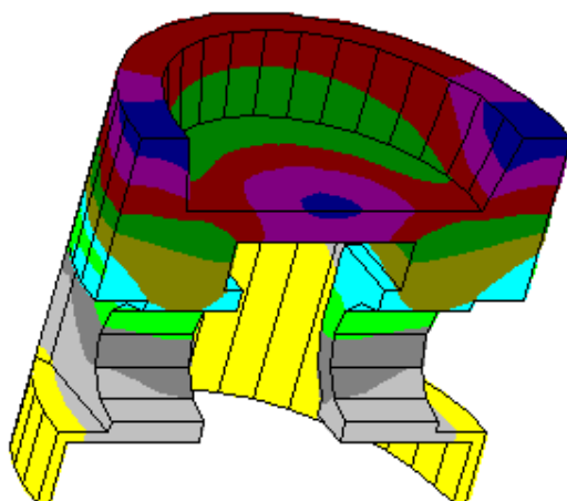
Рис. 7 Вид КОНСТРУКЦИИ при Lbrv=2
